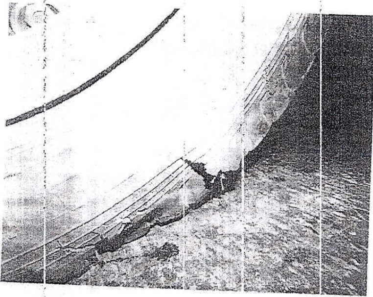
Fotografía n° 23: realizada a los daños de la rueda antes mencionada, aproximación y desde otro ángulo fotográfico -
