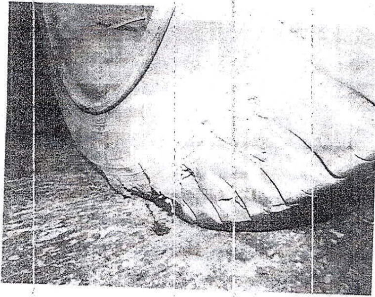
Fotografía n° 22: realizada a la rueda trasera dual externa izquierda del carro de la "rastra", se observan daños en la misma.-
