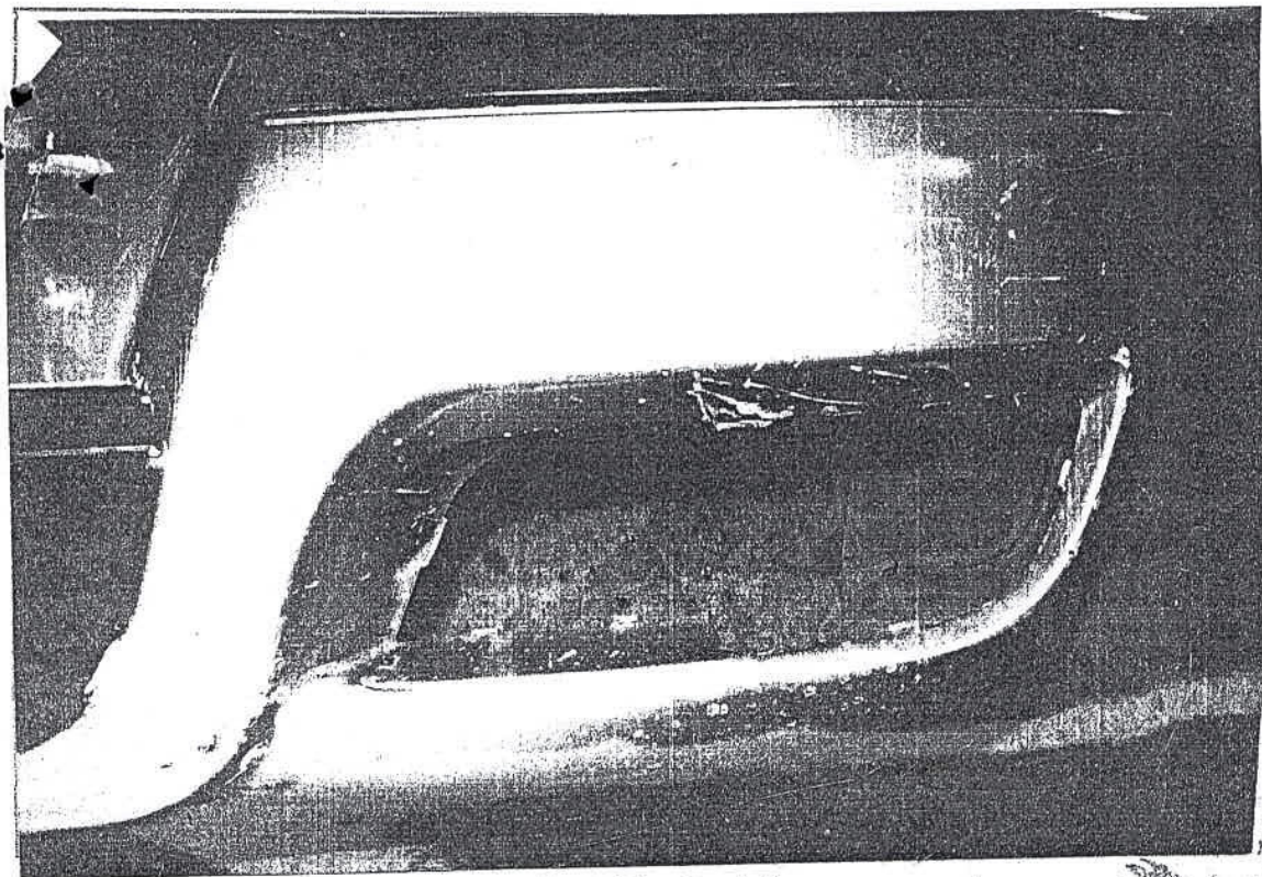
Fotografía n° 21: Toma en aproximación de daño en paragolpe.
