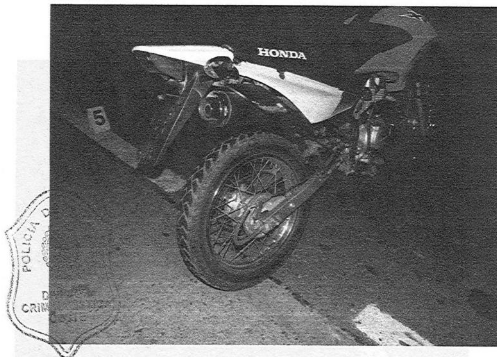
FOTOGRAFIA N° 34: Toma al lateral derecho parte de atrás de la motocicleta se observa daños en el cubre escape guiño y extremo del escape.-
