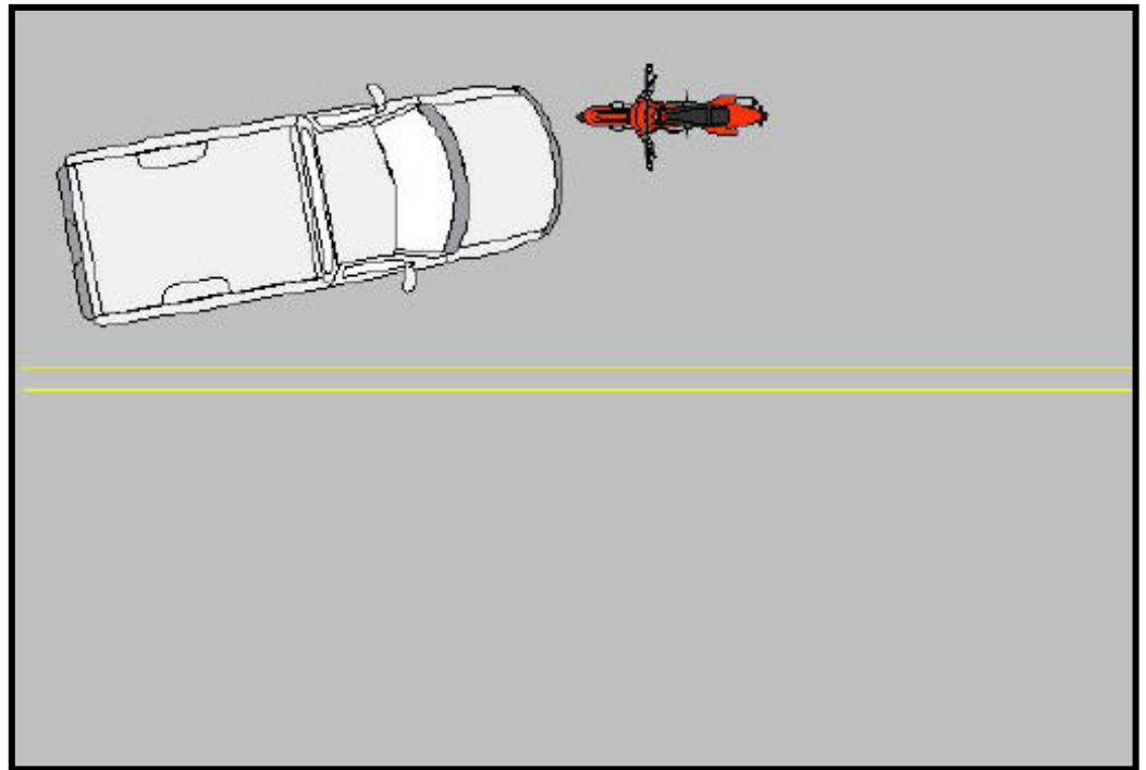
Grafico Nro.4: Se ilustra la forma de contacto entre ambos rodados, se denomina Colisión Frontal angular ya que ambos colisionan con la parte frontal, donde los ejes longitudinales de cada vehículo forman un ángulo inferior a 90^\circ .
