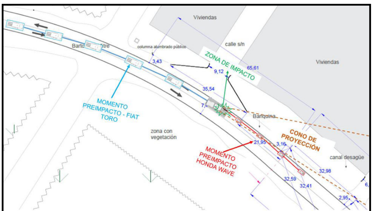
Grafico Nro.5: Se ilustra los momentos previo al impacto entre los vehículos, se señala la zona de impacto y se grafica el cono de proyección.
