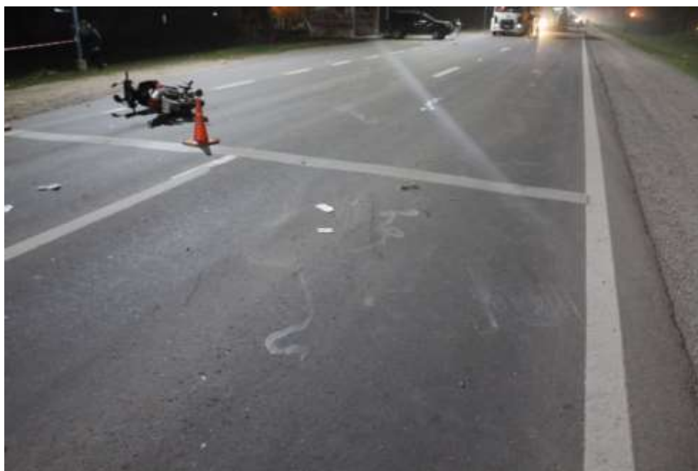
Fotografía n° 11: Panorámica de Sur a Norte, por carril Este de la Ruta antes mencionada, donde se observa marca de arrastre. -
